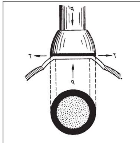
Рис. 2.19. Тонometr Маклакова
